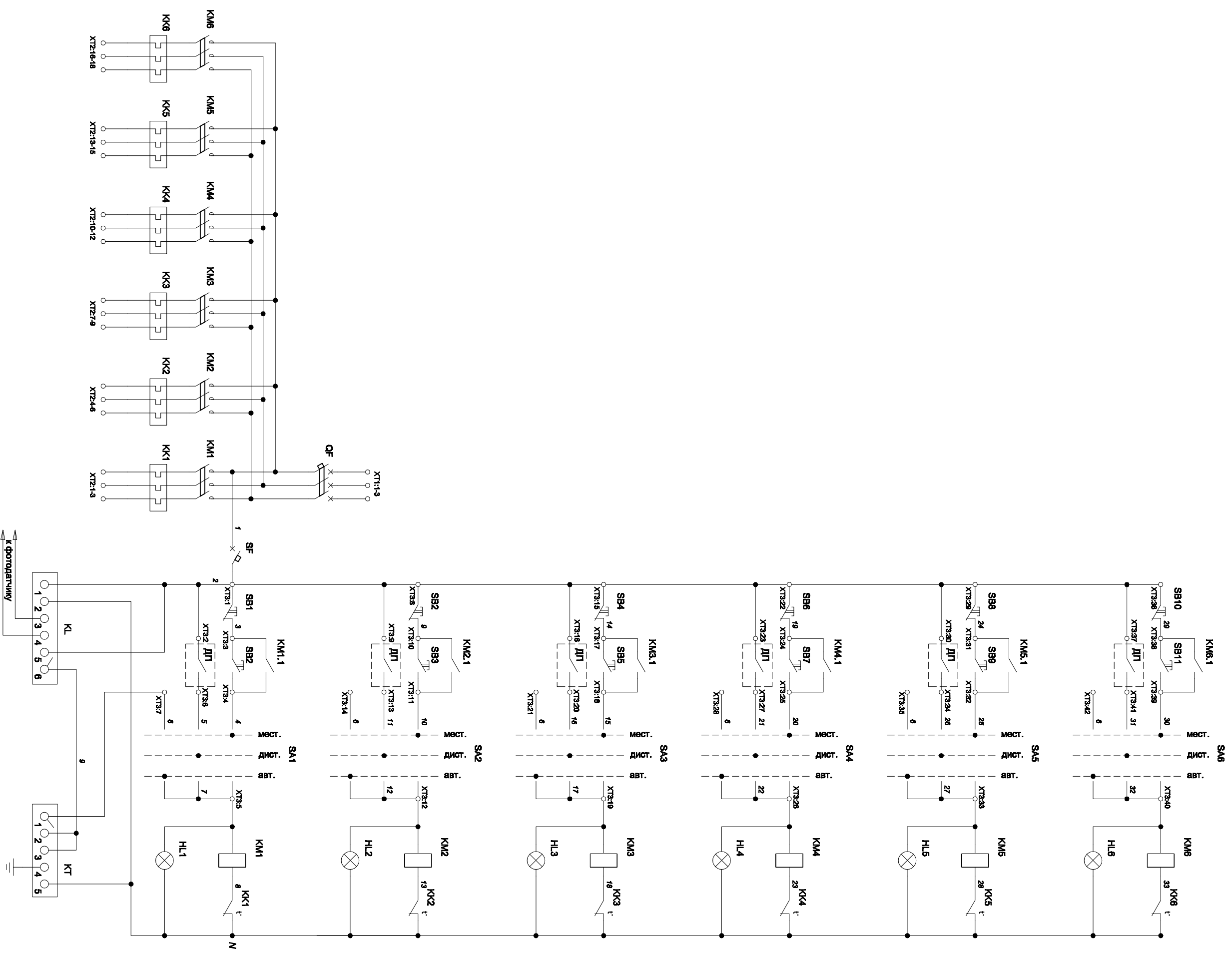
Принципиальная электрическая схема ЯУО 9601 (ШР-1006-А-1Р31)
