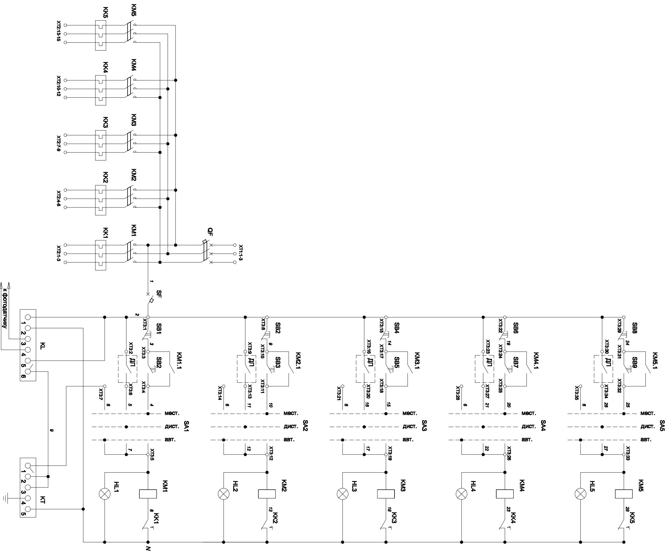
Принципиальная электрическая схема ЯУО 9601 (ЦР-1005-А-ІР31)
